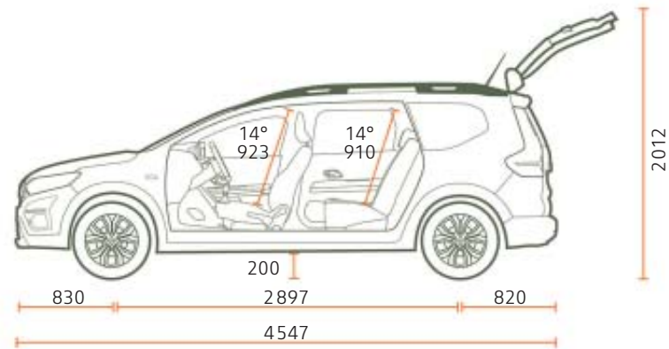
ZIJAAANZICHT 5 ZITPLAATSEN
