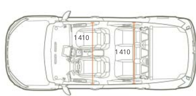
BOVENAANZICHT 5 ZITPLAATSEN
